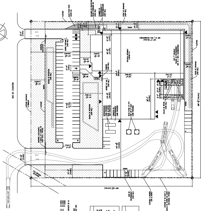
1. PLAN D'IMPLANTATION 1/200
